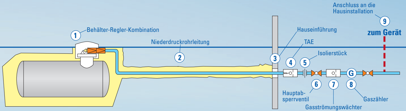
Erdgedeckte Versorgungsanlage mit Hauseinführung
